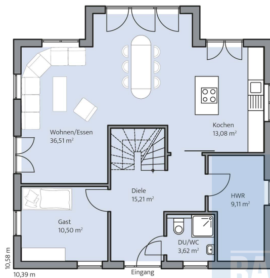
Haus Meinke Grundriss
