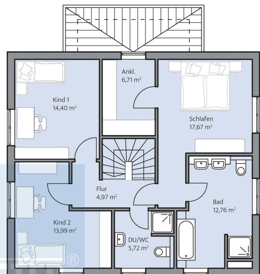
Haus Meinke Grundriss
